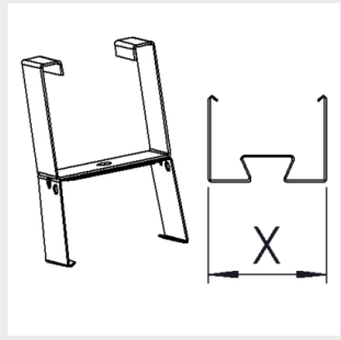
3508173 Gamma Eco S riputuskiskokannake 110 (7)
