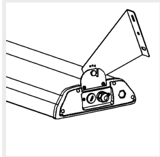
Säädettävä seinäkannake
