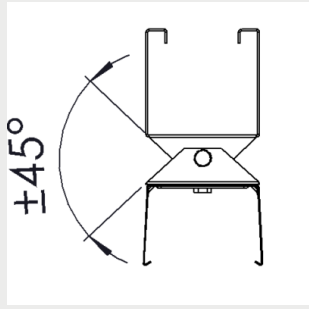
Säädettyvä valaisinkiskokannake
