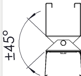
9905201 Gamma Eco S säädettävä ripustuskiskokannake 120
