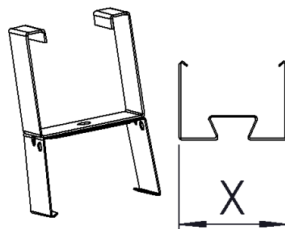
3508172 Gamma/Eco S ripustuskiskokannake 82
