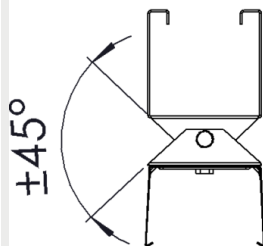
9905200 Gamma/Eco S säädettävä ripustuskiskokannake 70
