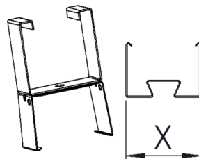
3508173 Gamma/Eco S ripustuskiskokannake 120
