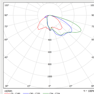
SIRIUS S 08 1v1 Upp till 40W
