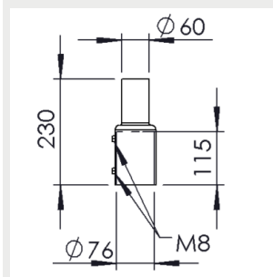
5205037 Röradapter 76mm -> 60mm
