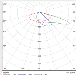
SIRIUS S 01 1v1 Upp till 40 W
