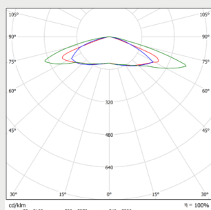
SIRIUS S 09 1v1 Upp till 40W
