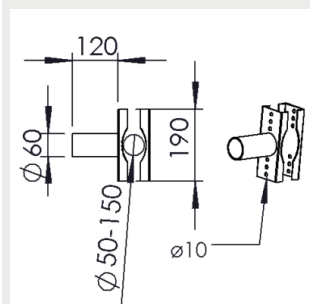
3608220 Rörfäste
