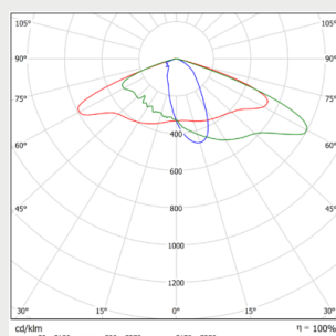
SIRIUS S S02 1v1
