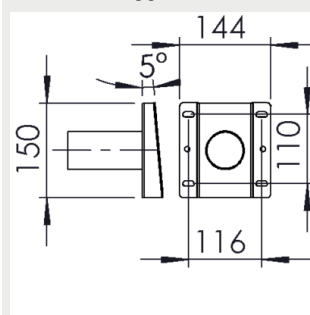
3608061 Väggfäste
