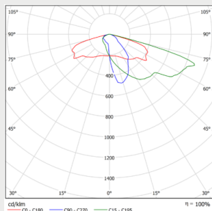
SIRIUS S 02 1v1 Upp till 40 W
