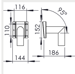
3608101 Takfäste
