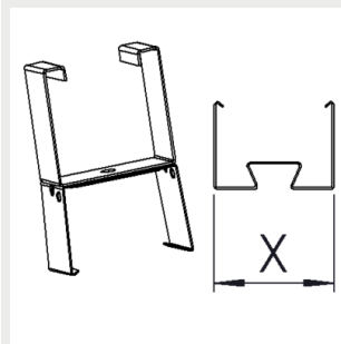
3508171 Gamma Eco S skenfäste 70 (7)
