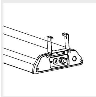
9905223 Sigma skenfäste 110
