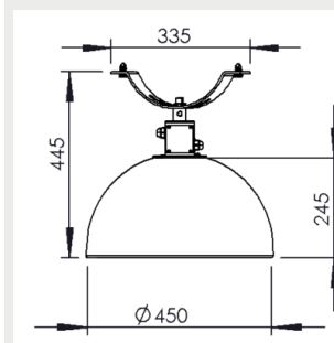
Tråd monterings dimensioner
