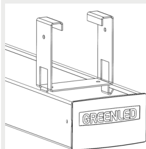
9908435 Skenfäste MEK 70
