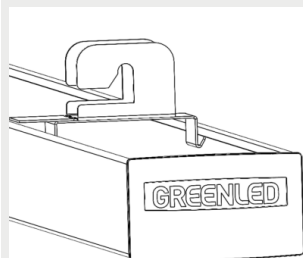
3508103 Horizontal vajerfäste max 8 mm
