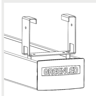
E1500147 Skenfäste MEK 82 vit
