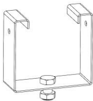
E 1500223 Origi MEK 70 End cap bracket
