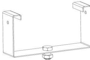
E 1500225 Origi MEK 110 End cap bracket
