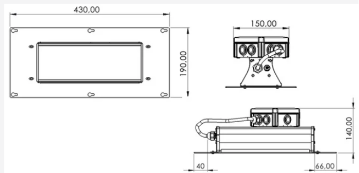
E1500278 Origi Canopy mini recessed frame
